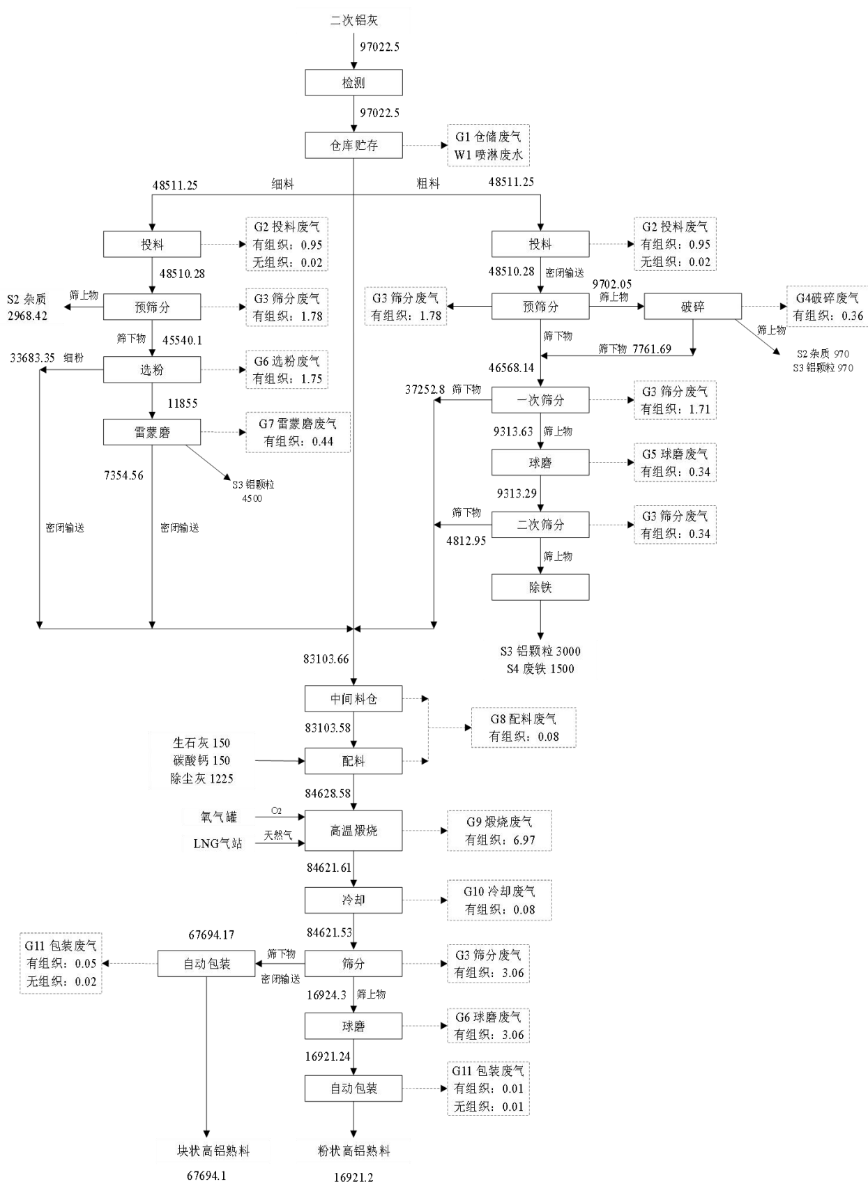
图1.4-5 变更后项目物料平衡图
