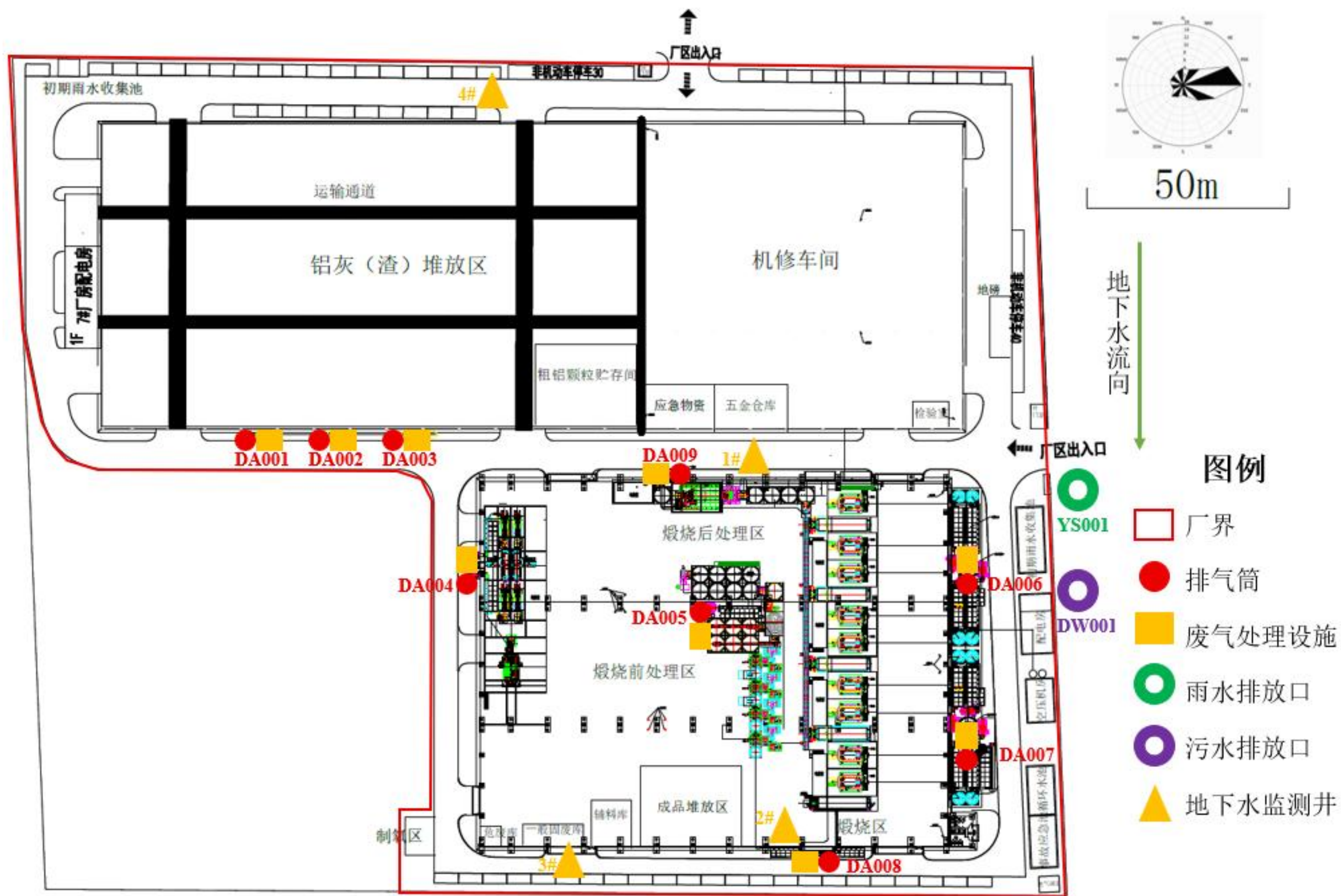
图 1.4-2 本次变更后车间平面布置图
