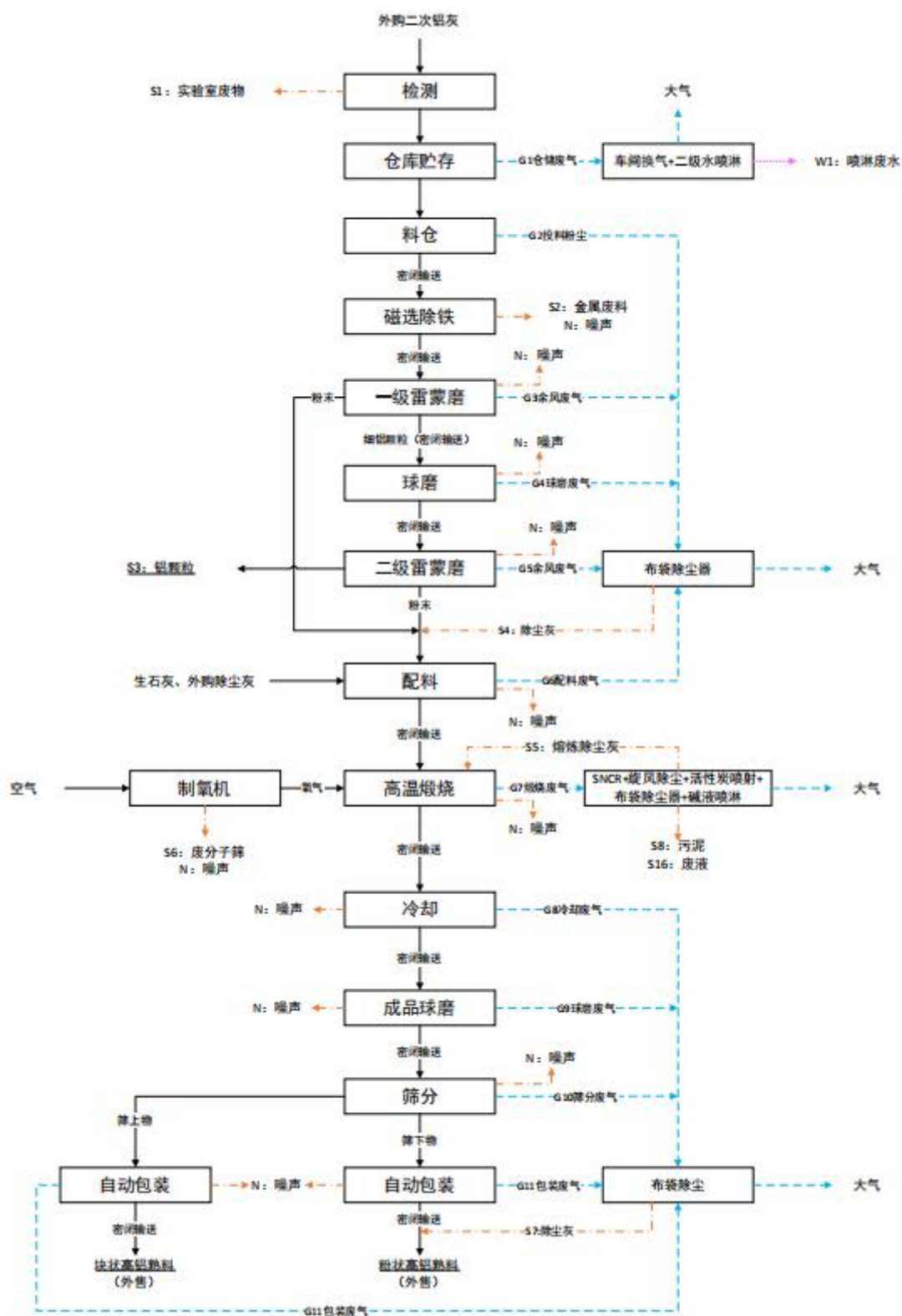
图 1.4-3 环评中生产工艺流程图
