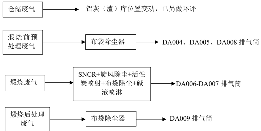
图 4-1 废气收集处理示意图
