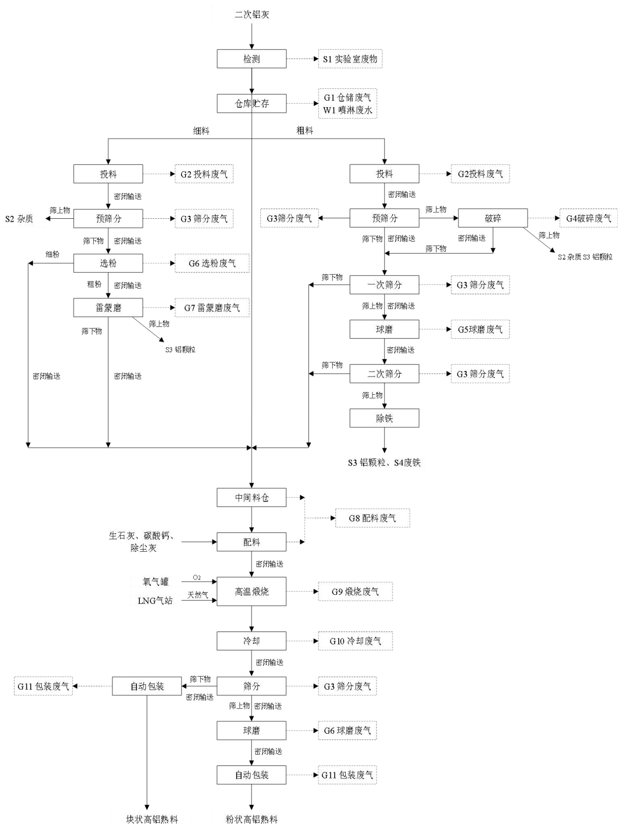
图 1.4-4 变更后生产工艺流程图
